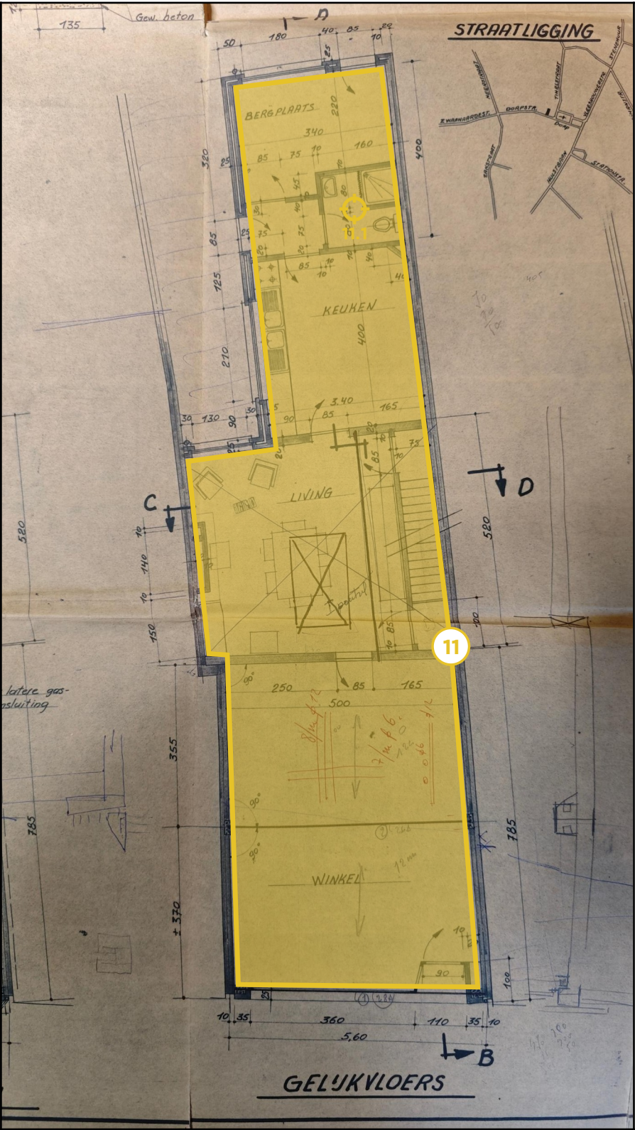
Legende van plan 1.3: Gelijkvloers: plafonds
